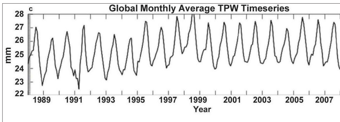
Figuur 4.15: Trend in Total Precipitable Water vapor. Bron: NASA. 100
