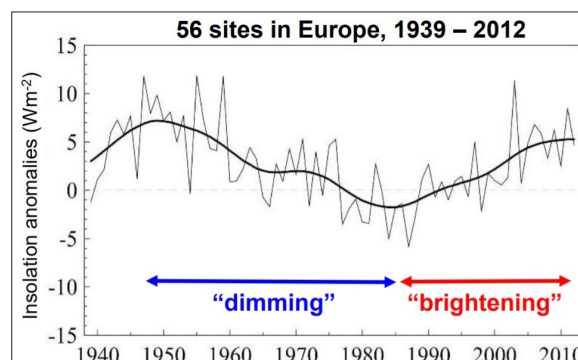
Figuur 3.6: Relatieve veranderingen van gemeten zonnestraling aan het oppervlakte. Bron: Martin Wild, AGU Fall presentatie 2015.
