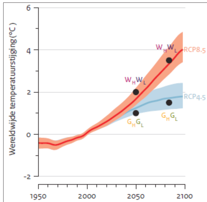
Figuur 3.1: Klimaatscenario's van het KNMI voor 2050 en 2085 ten opzichte van de mondiale scenario's van het IPCC. Twee uitstootscenario's: RCP4.5 (stabilisatie) en RCP8.5 (hoge uitstoot). Gelekleurde banden: spreiding tussen klimaatmodellen; lijnen: gemiddelde over de modellen; Punten: wereldwijde temperatuurstijging zoals toegepast in de KNMI'14-klimaatscenario's voor Nederland. 45
