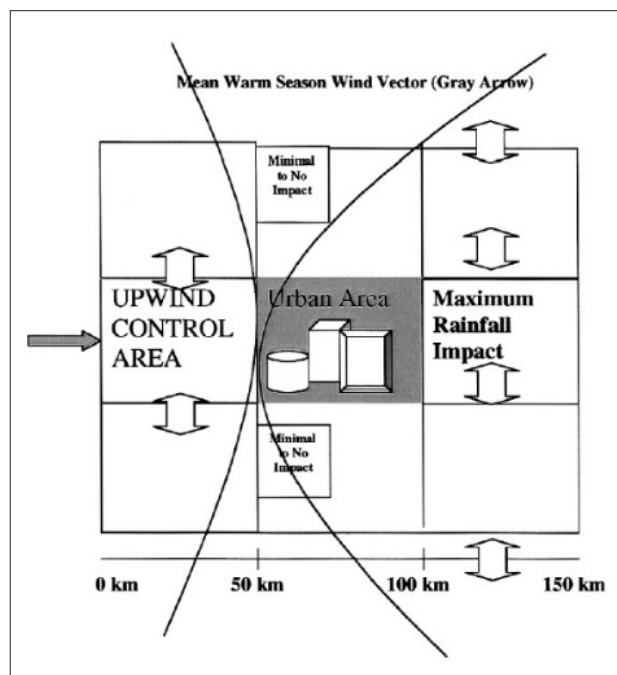
Figuur 4.23: Schematische weergave van het impactgebied van neerslag als gevolg van UHI. Bron: Shepherd et al.
