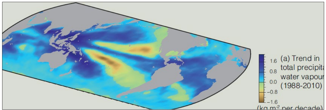
Figuur 4.14: Trend beschikbare waterdamp boven oceanen in \text{kg}/\text{m}^2 . Bron: IPCC AR5 WG1. 98
