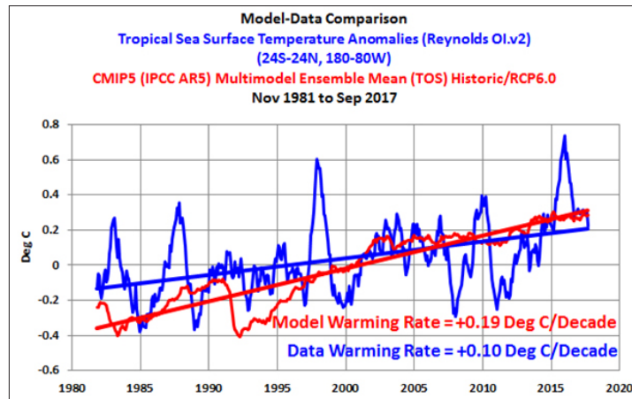
Figuur 2.25: Opwarming in het oostelijke deel van de Grote Oceaan, modellen versus waarnemingen.
