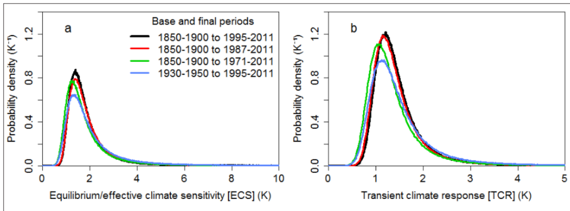
Figuur 2.3: observationele schattingen voor ECS en TCR op basis van gegevens uit het vijfde IPCC-rapport.
