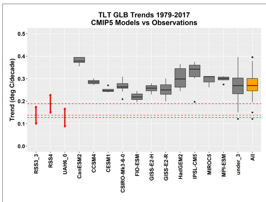
Figuur 2.14: Waargenomen mondiale temperatuurtrend in de lagere troposfeer versus trends in de modellen voor de periode 1979-2017. Helemaal rechts in geel het gemiddelde van alle modellen. Er zijn twee versies van RSS getoond omdat de meest recente versie aanzienlijk afwijkt van de vorige versie. Bron: Climate Audit. 19
