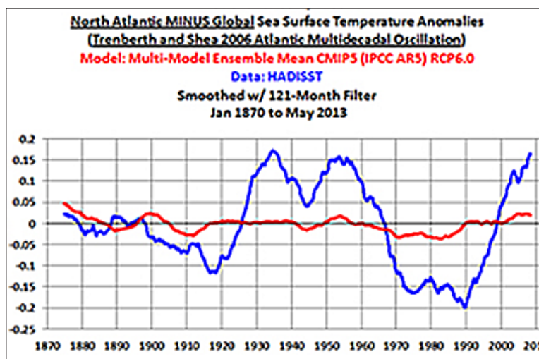
Figuur 2.9: De temperatuur in de Noord-Atlantische Oceaan minus de mondiale zeewatertemperatuur. In blauw waarnemingen, in rood modellen. Het modelgemiddelde pikt het AMO-sigitaal duidelijk niet op. Bron: Bob Tisdale.
