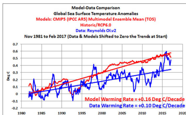
Figuur 2.24: Opwarming van de oceanen, modellen versus waarnemingen. Bron: Bob Tisdale.
